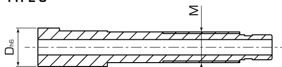
TIPO 3 TYPE 3
